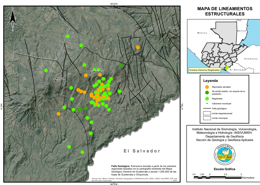
Figura 2: Mapa de los eventos sísmicos registrados
