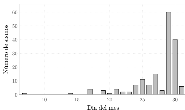
Figura 1: Histograma con los eventos sísmicos registrados
