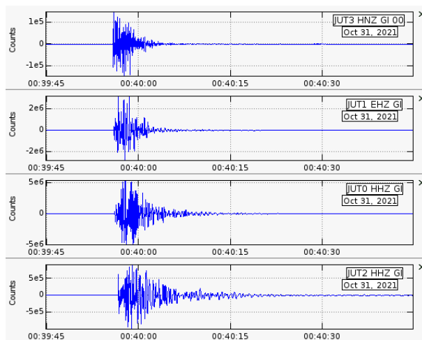
Figura 3: Sismograma de las estaciones temporales
