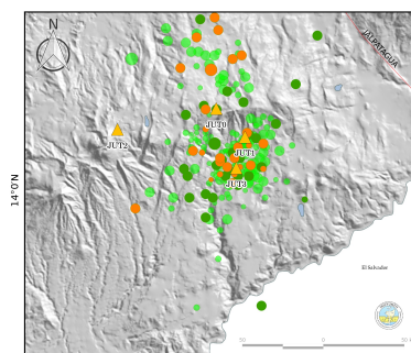
(c) Dispersión de las profundidades de los sismos registrado
