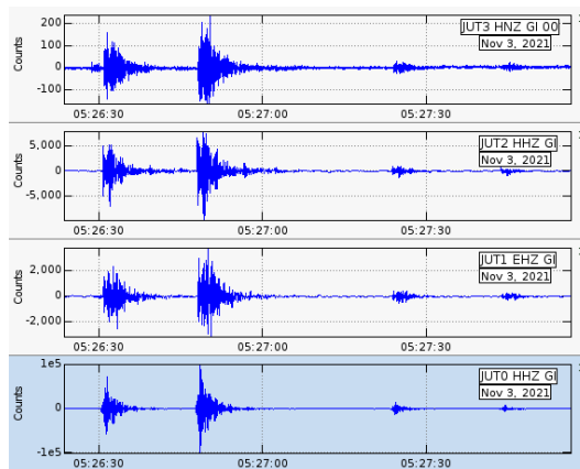
(b) Sismograma de las estaciones temporales instaladas
