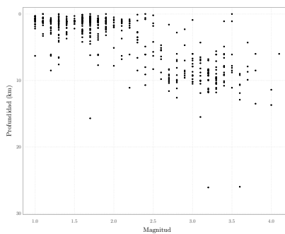
(c) Dispersión de las profundidades de los sismos registrado
