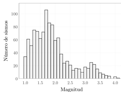
(b) Histograma de las magnitudes de los sismos registrados
