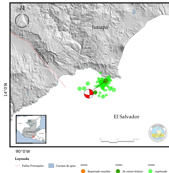
Figura 1: Mapa de los eventos sísmicos registrados
