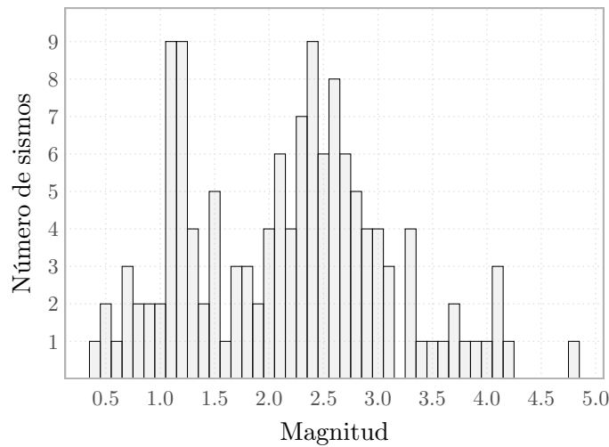
Figura 3: Distribución de las magnitudes de los 134 eventos sísmicos registrados durante la semana.
