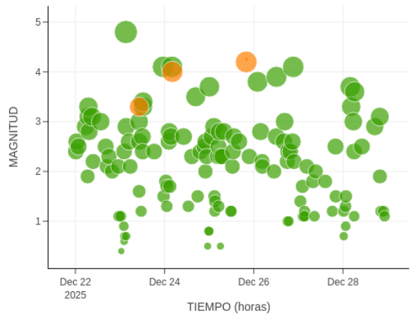
Figura 2: Distribución temporal de los 134 eventos sísmicos registrados durante la semana.
