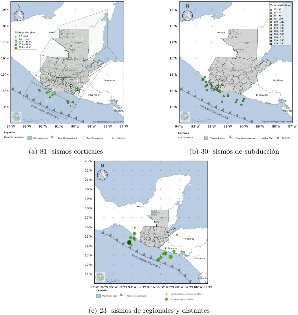
Figura 4: Clasificación de los 134 eventos sísmicos según su fuente sísmica
