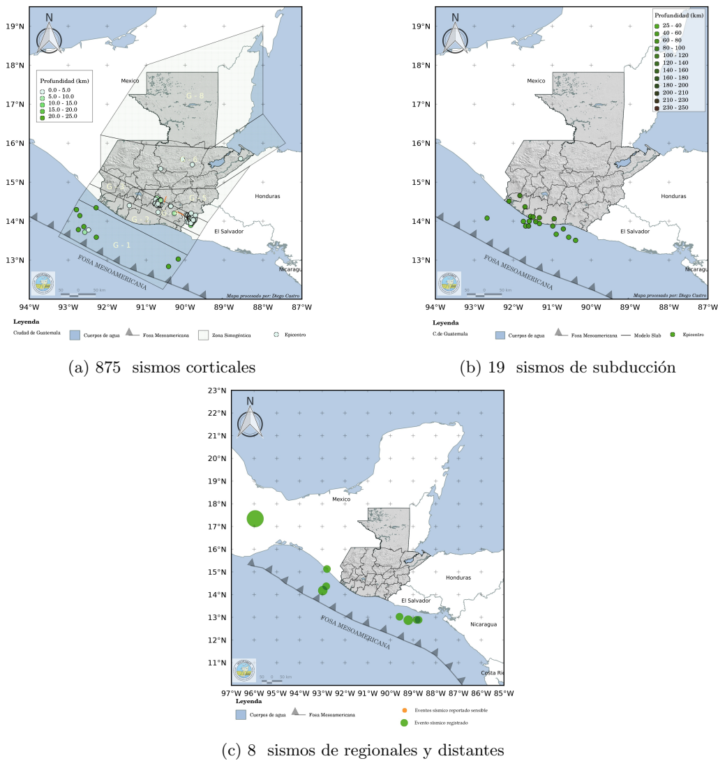
Figura 4: Clasificación de los 902 eventos sísmicos según su fuente sísmica
