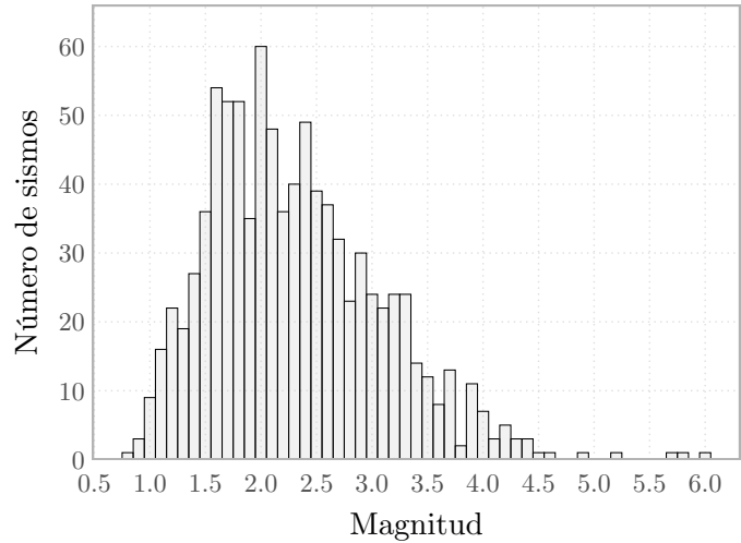
Figura 3: Distribución de las magnitudes de los 902 eventos sísmicos registrados durante la semana.
