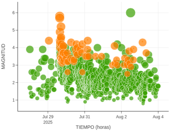
Figura 2: Distribución temporal de los 902 eventos sísmicos registrados durante la semana.
