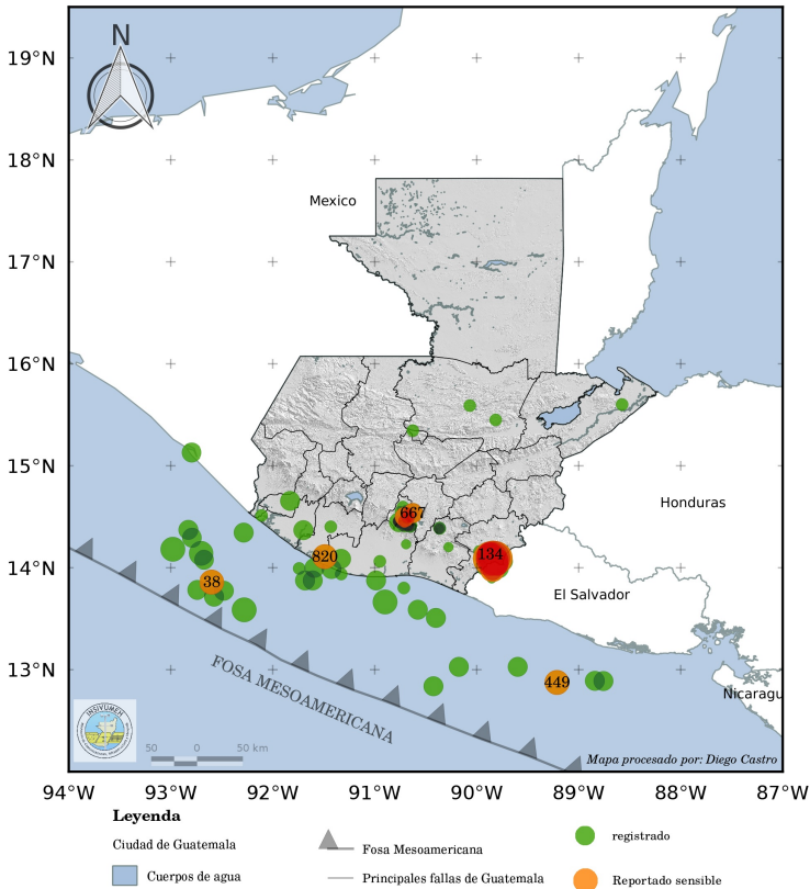
Figura 1: Localización geográfica de los 902 eventos sísmicos registrados durante la semana.
