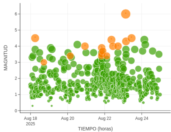
Figura 2: Distribución temporal de los 597 eventos sísmicos registrados durante la semana.
