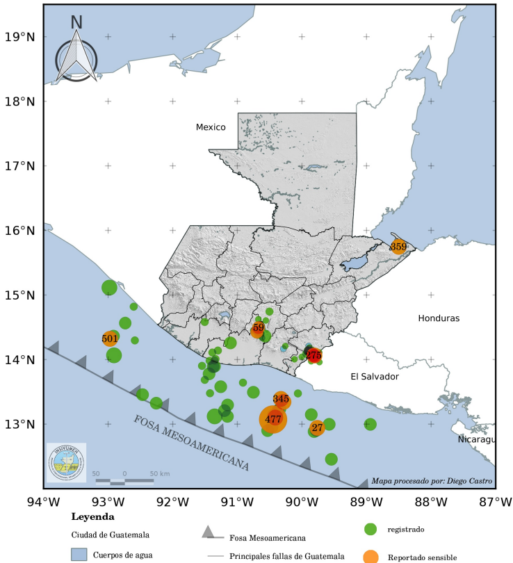
Figura 1: Localización geográfica de los 597 eventos sísmicos registrados durante la semana.
