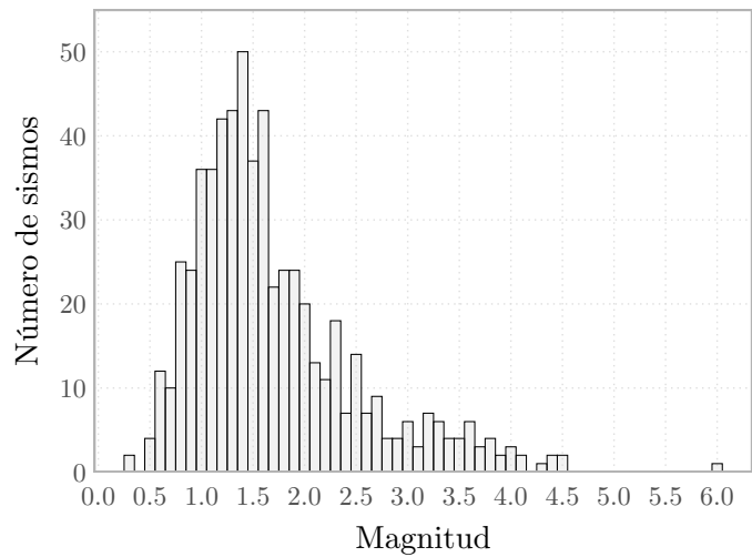
Figura 3: Distribución de las magnitudes de los 597 eventos sísmicos registrados durante la semana.
