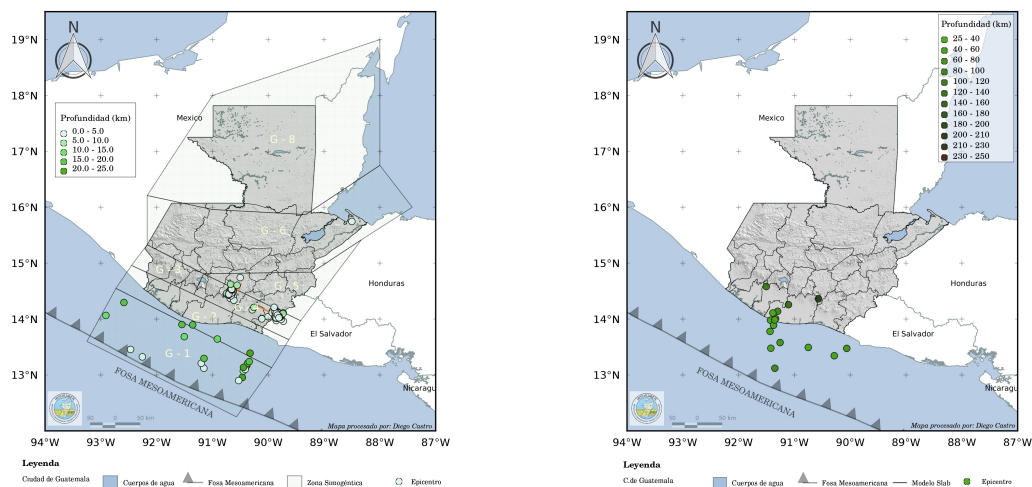
(a) 568 sismos corticales (b) 16 sismos de subducción
