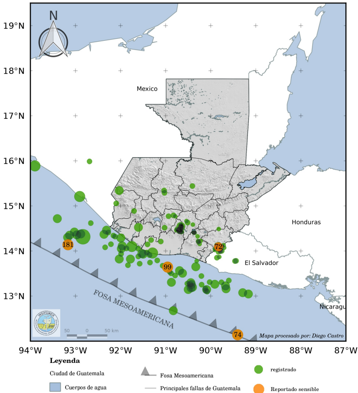
Figura 1: Localización geográfica de los 222 eventos sísmicos registrados durante la semana.
