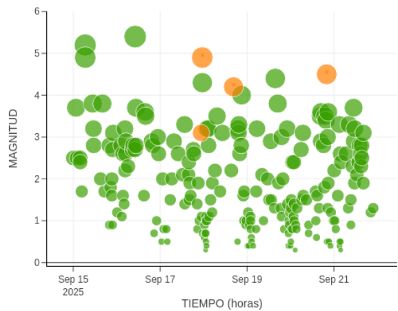
Figura 2: Distribución temporal de los 222 eventos sísmicos registrados durante la semana.
