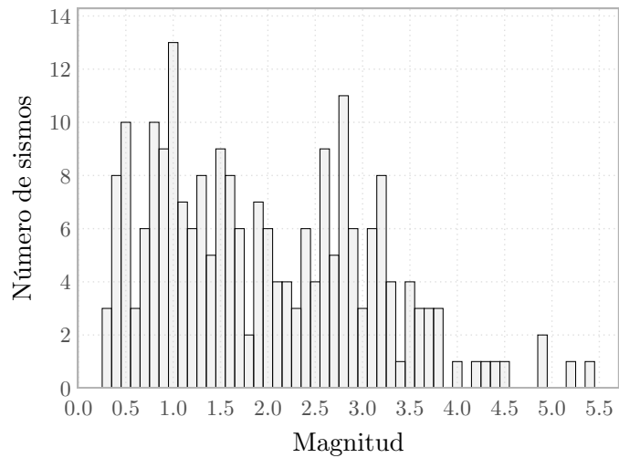
Figura 3: Distribución de las magnitudes de los 222 eventos sísmicos registrados durante la semana.
