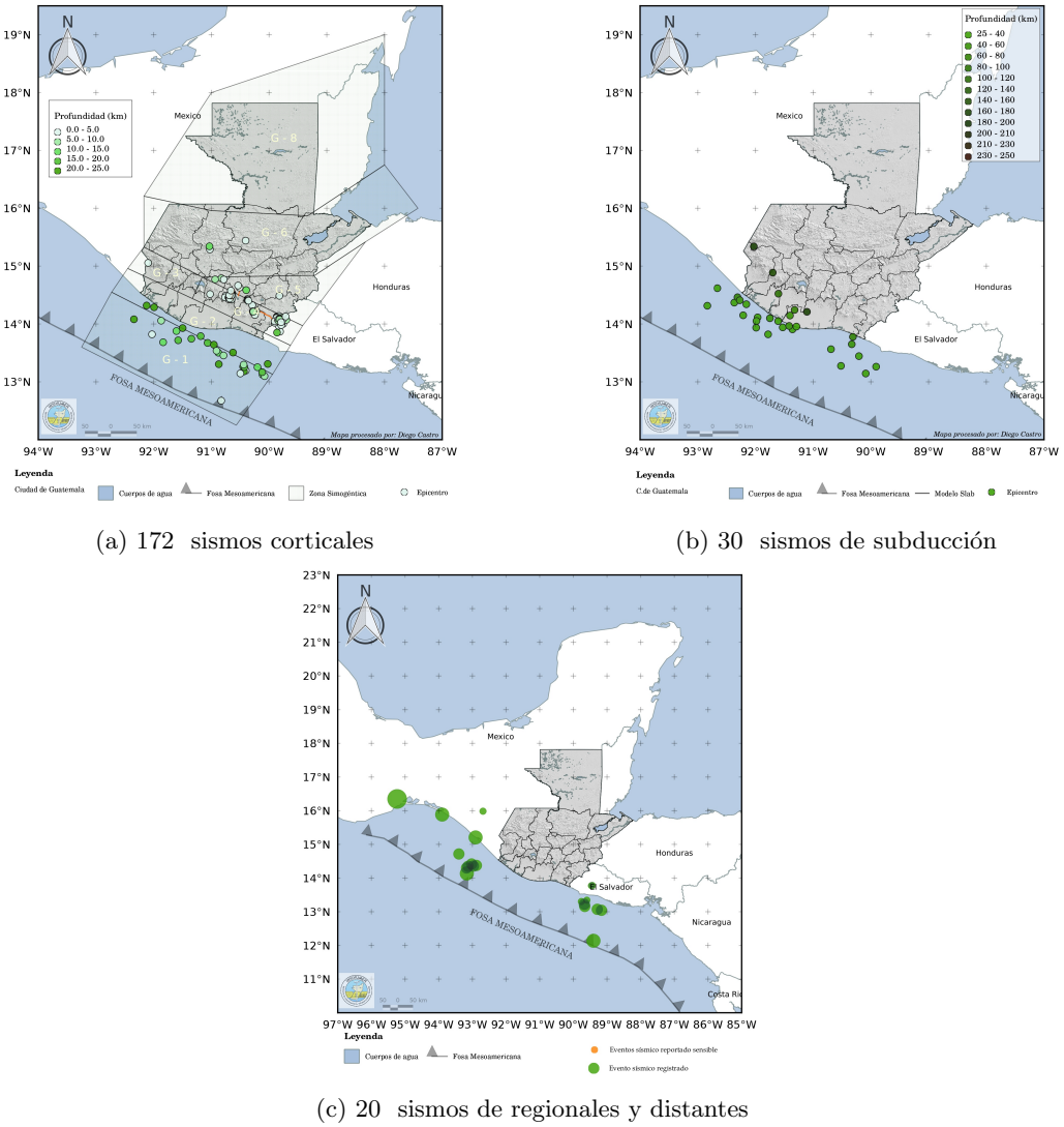
Figura 4: Clasificación de los 222 eventos sísmicos según su fuente sísmica
